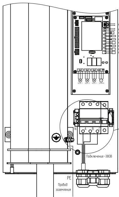
Рис. 3 Схема подключения электроводонагревателя
