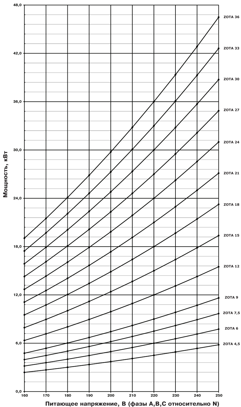
Рис.11 График изменения мощности электроводонагревателя в зависимости от питающего напряжения
