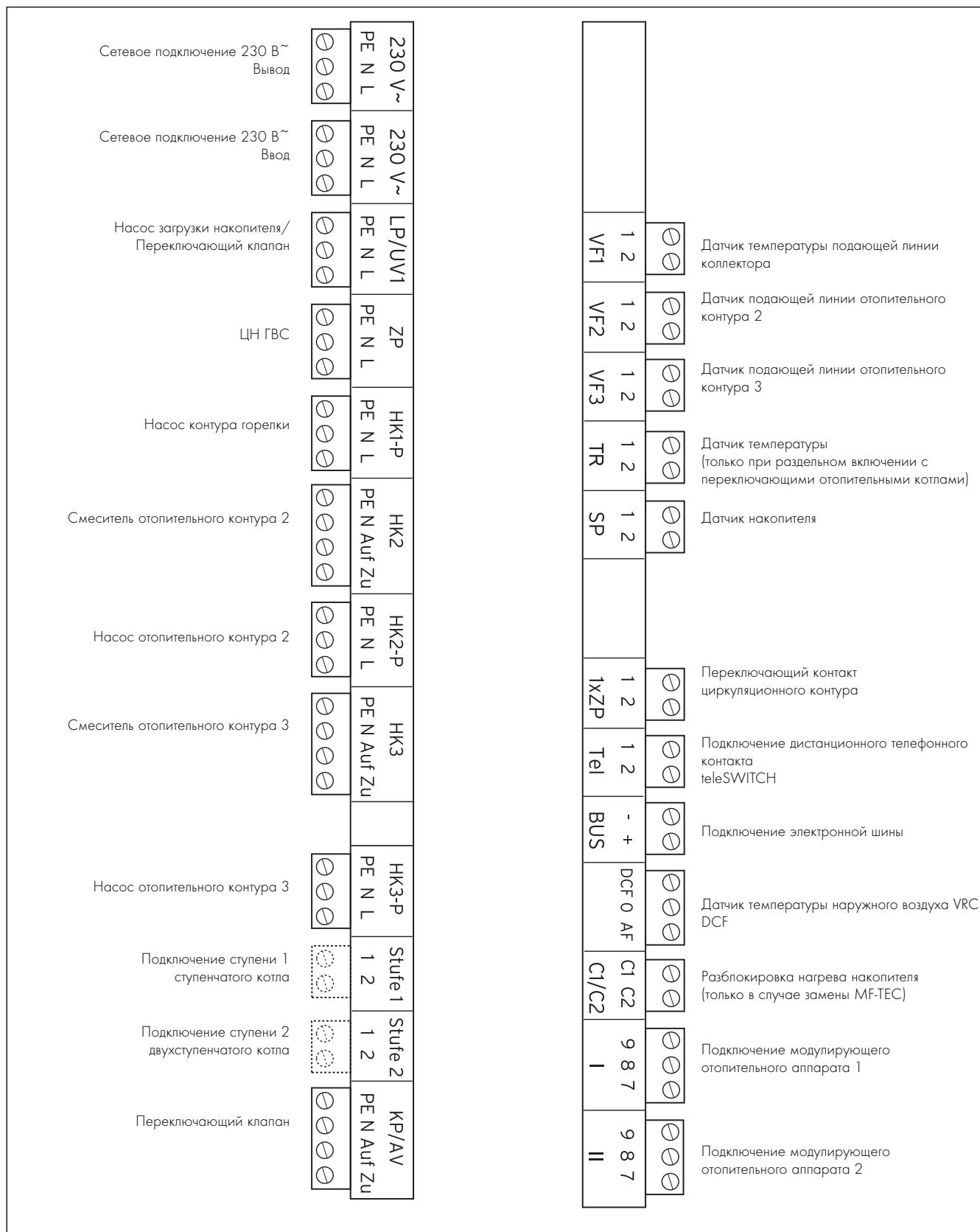
Рис. 5.4 Клеммная колодка
