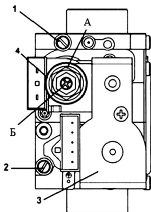
Рис. 11. Регулятор газа Sit 845 Sigma
