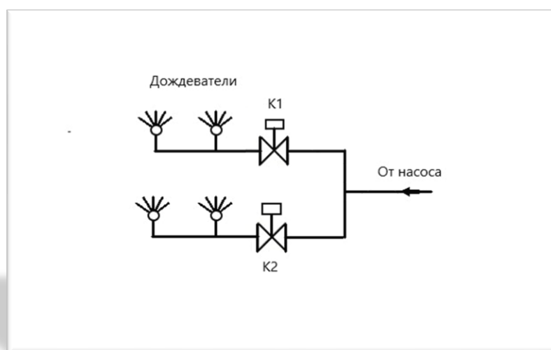
Рисунок А1 – Схема автополива без емкости
