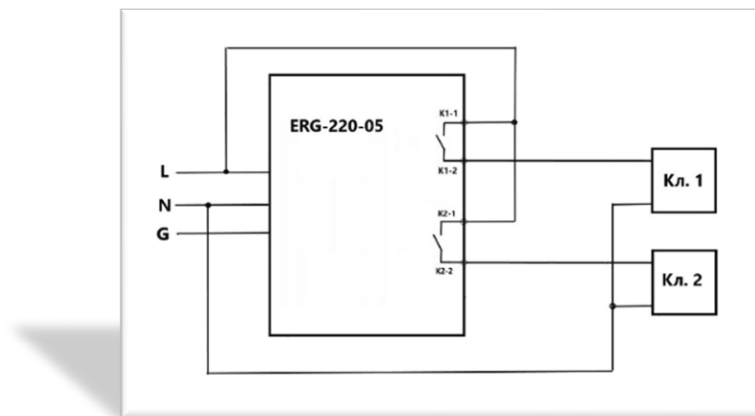
Рисунок А5 – Схема подключения электромагнитных клапанов
