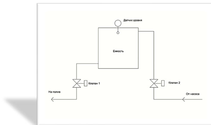
Рисунок А3 – Схема капельного полива с емкостью
