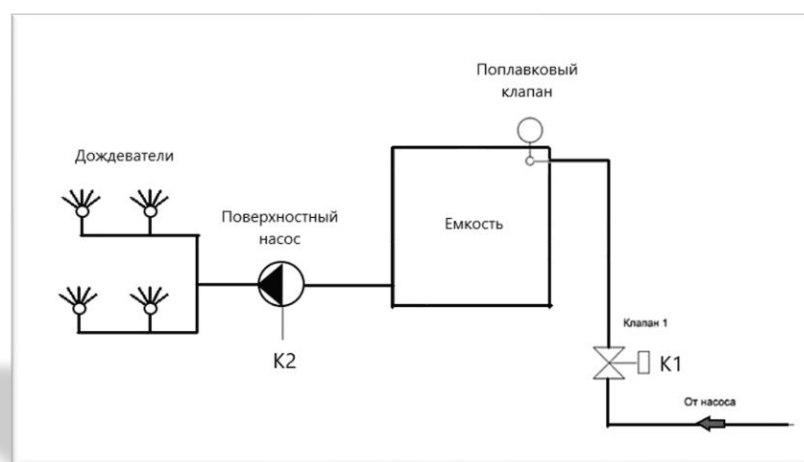
Рисунок А2 – Схема автополива с емкостью
