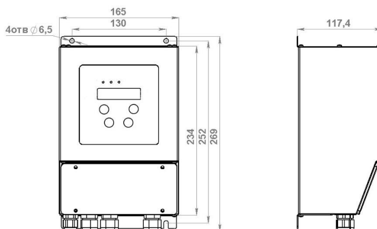
Рисунок 14 – Габаритные и установочные размеры ПЧ
