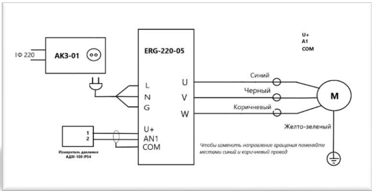
Рисунок 5в – Схема подключения ПЧ к трехфазному насосу 220 В
