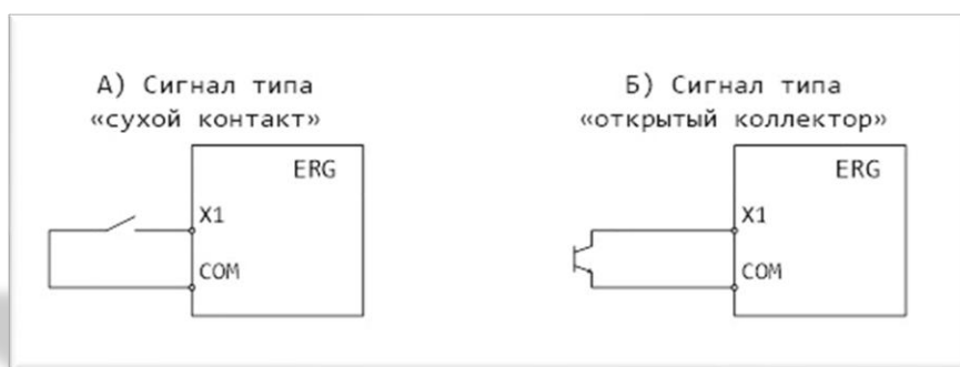
Рисунок А4 – Схема подключения датчика уровня
