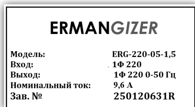
Рисунок 3 – Шильдик изделия
