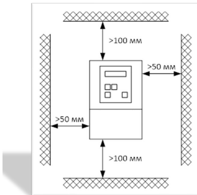
Рисунок 4 – Установка ПЧ
