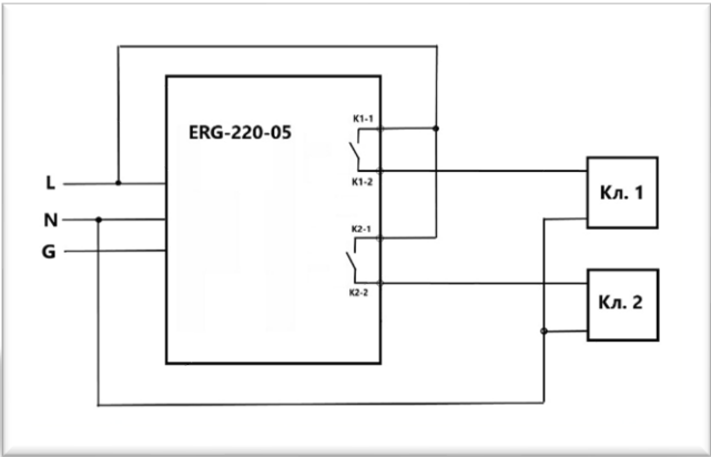
Рисунок 10 – Подключение электромагнитных клапанов автополива
