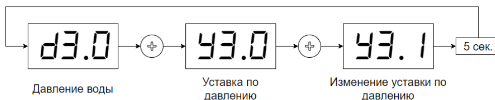
Рисунок 14 – Изменение уставки давления
