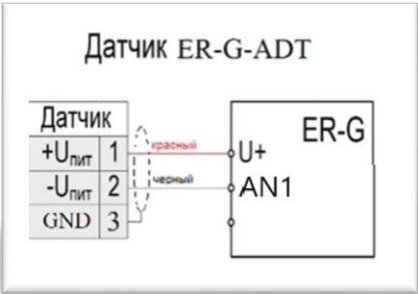
Рисунок 7 – Подключение датчика ER-G-ADT
