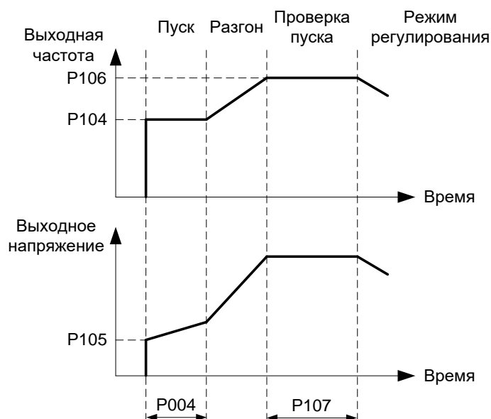
Рисунок 2 – Диаграмма работы ПЧ в режиме пуска
