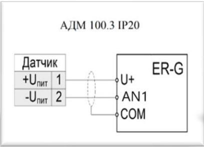
Рисунок 8 – Схемы подключения датчика давления АДМ-100 в корпусе IP20 и IP54
