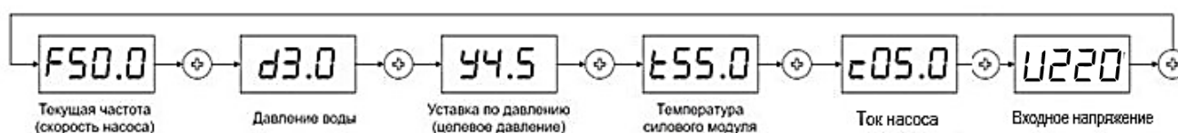
Рисунок 15 – Изменение параметров при P008=1
