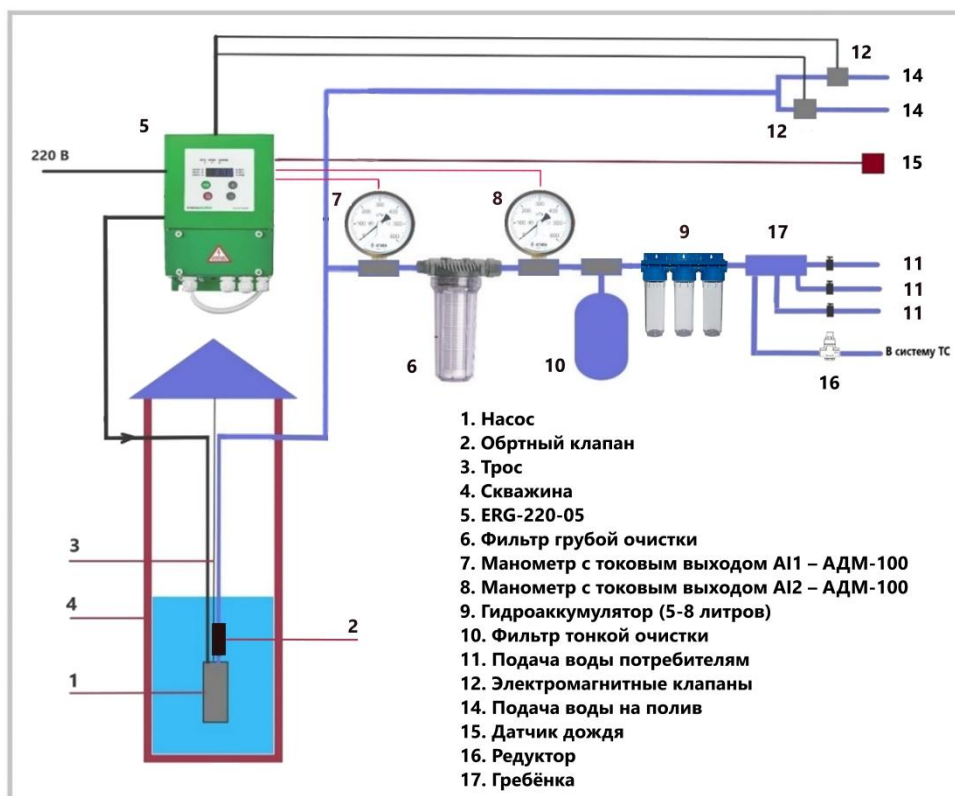
Рисунок 1 – Схема автоматизации системы водоснабжения
