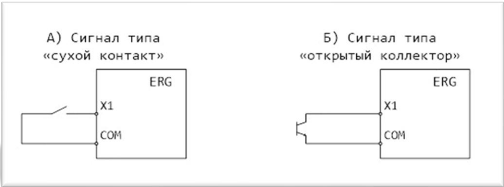
Рисунок 7 – Подключение датчика ER-G-ADT
