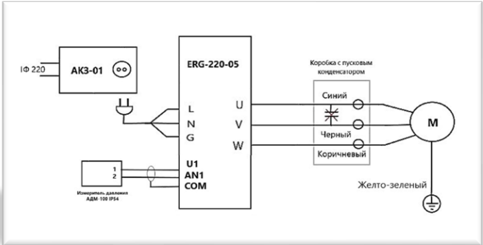
Рисунок 5б – Схема подключения ПЧ к двухфазному (бесконденсаторному) насосу на 220 В
