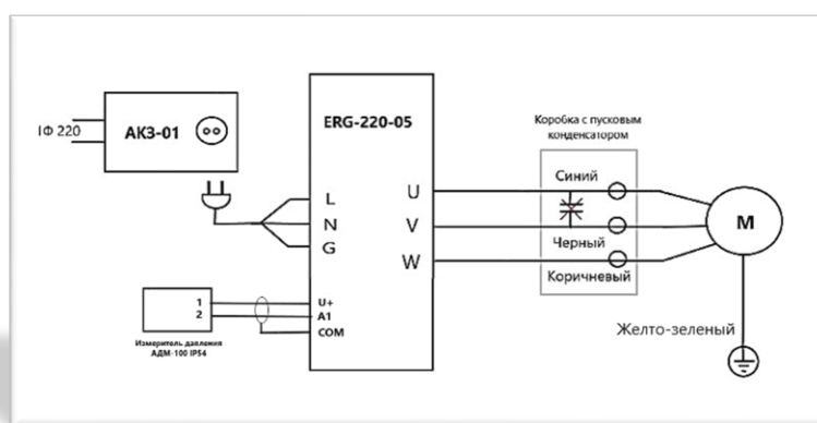
Рисунок Б1 – схема подключения насоса в двухфазном режиме
