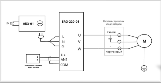
Рисунок 5а – Схема подключения ПЧ к однофазному насосу на 220 В
