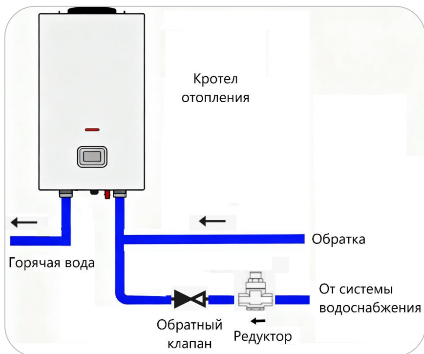
Рисунок В1 – условная схема подпитки системы теплоснабжения
