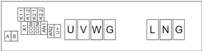
Рисунок 6 – Расположение клемм ПЧ
