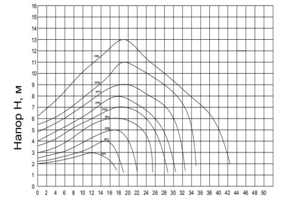
Производительность Q, м³/ч STAR PX3 PP1-PP9
