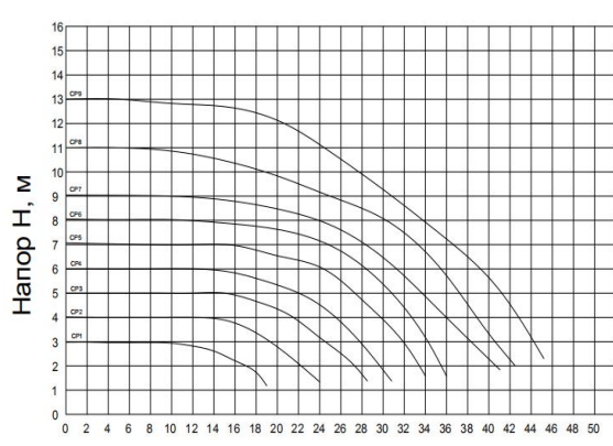
Производительность Q, м³/ч STAR PX3 CP1-CP9
