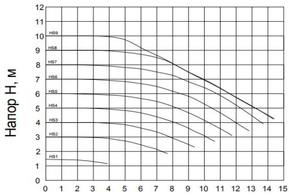
Производительность Q, м³/ч STAR PX1 HS1-HS9
