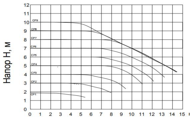
Производительность Q, м 3 /ч STAR PX1 CP1-CP9
