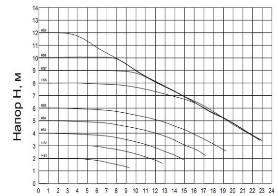
Производительность Q, м³/ч STAR PX2 HS1-HS9
