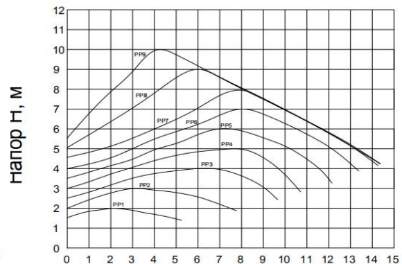
Производительность Q, м 3 /ч STAR PX1 PP1-PP9
