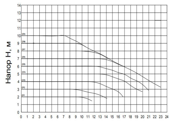
Производительность Q, м³/ч STAR PX2 CP1-CP9
