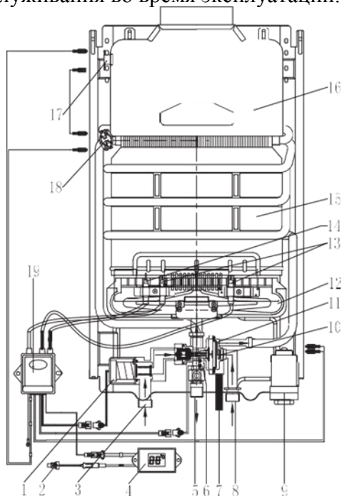
Рис. 1. проточный газовый водонагревательный аппарат "RISPA "
