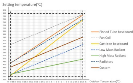
Настройка температуры обогрева помещения для управления наружным датчиком
