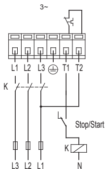
Рис. 9 Схема подключения трехфазного насоса при использовании внешнего механического пускателя ВКЛ/ВЫКЛ
