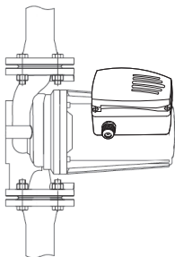
Рис. 2 Допустимое расположение вала насоса
