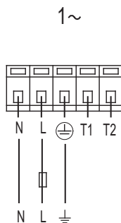
Рис. 10 Схема подключения однофазного насоса
