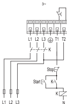
Рис. 8 Схема подключения трехфазного насоса при использовании внешнего электромагнитного пускателя ВКЛ/ВЫКЛ
