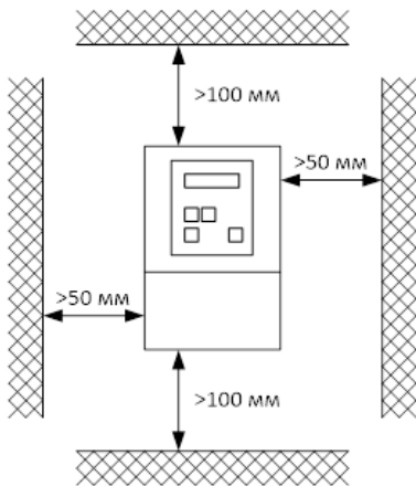
Рисунок 3 – Установка ПЧ
