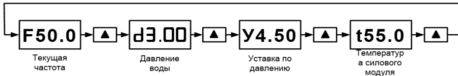
Рисунок 15 – Последовательность просмотра текущих параметров
