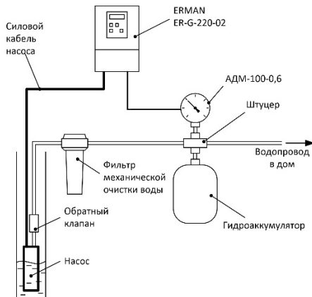
Рисунок 1 – Схема автоматизации системы водоснабжения
