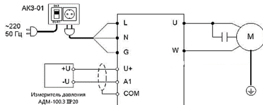
Рис 7а - Схема с измерителем АДМ-100.3 IP20 или аналогичным
