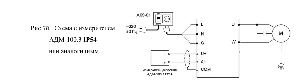
Рисунок 7 – Схемы подключения датчика давления АДМ-100 в корпусе IP20 и IP54
