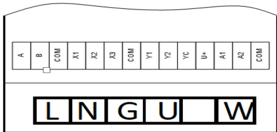
Рисунок 5 – Расположение клемм ПЧ
