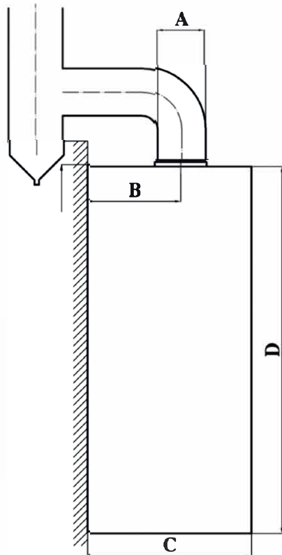
Рис. 17. Габаритные размеры
