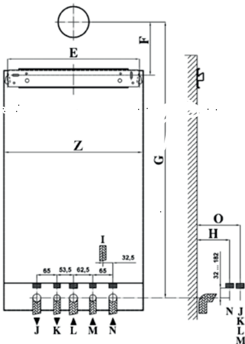
Рис. 18. Подключения
