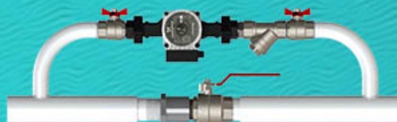
Байпасный узел в сборе
